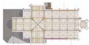
Charpentes
