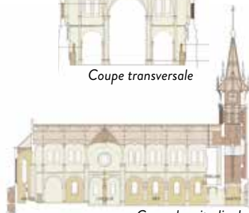
Coupe longitudinale
